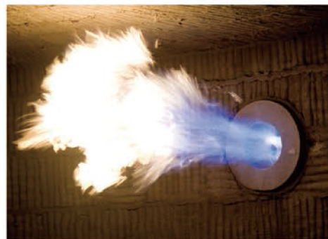
Flammenbild während der Aufheizphase. Nach Erreichen der Betriebs- temperatur > 850°C werden die Brenner zum Erreichen niedriger NOx-Werte flammenlos betrieben. To ensure lowest NOx- emissions the burners will be switched to flameless mode above 850°C.
